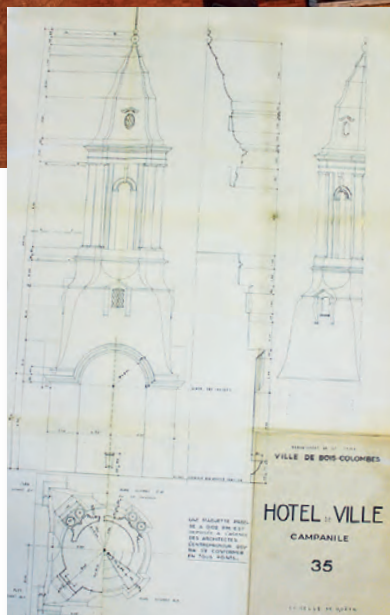
Le plan d'élévation du campanile des architectes E. Berthelot et G. Bovet, vers 1934-1935.
